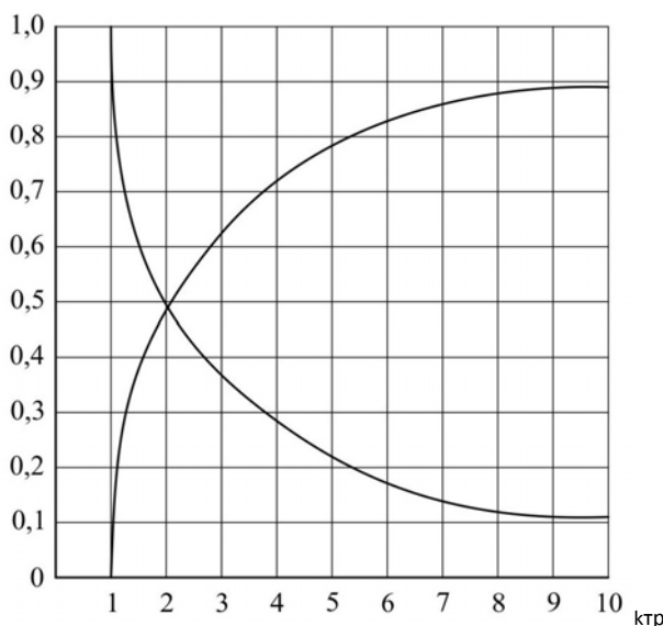
Рис. 1. Зависимость коэффициента использования силовых тиристоров и обратных диодов от коэффициента трансформации
