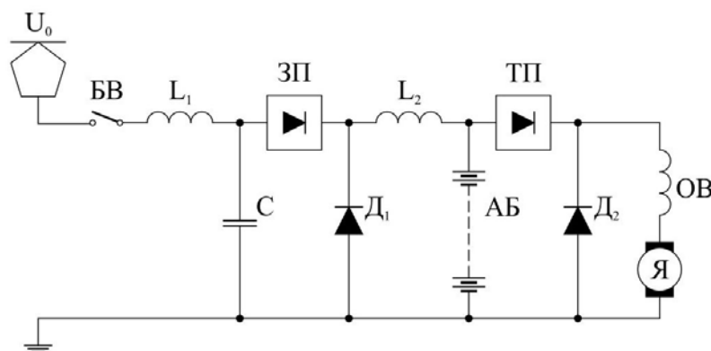
Рис. 3. Блок-схема комбинированного ЭПС с последовательным включением зарядного (ЗП) и тягового (ТП) ТИП
