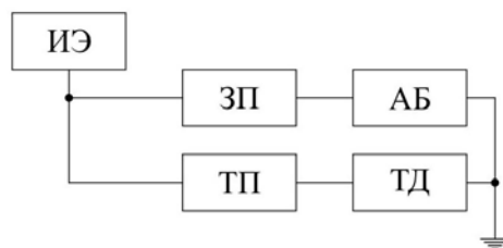
Рис. 2. Блок-схема комбинированного ЭПС с параллельным включением зарядного и тягового ТИП
